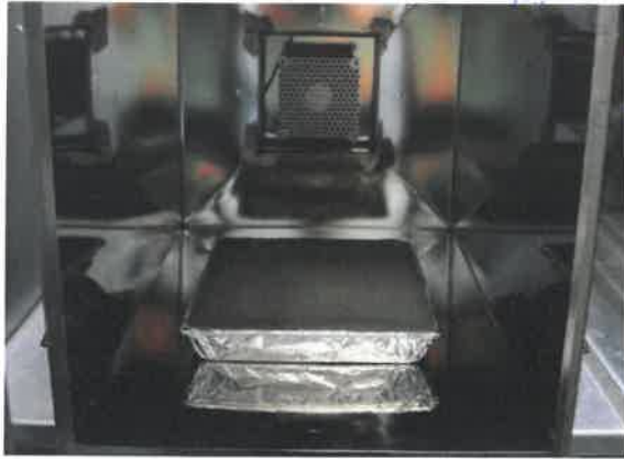
Bild 3: Prüfstück in der 200 L Emissionsprüfkammer.
